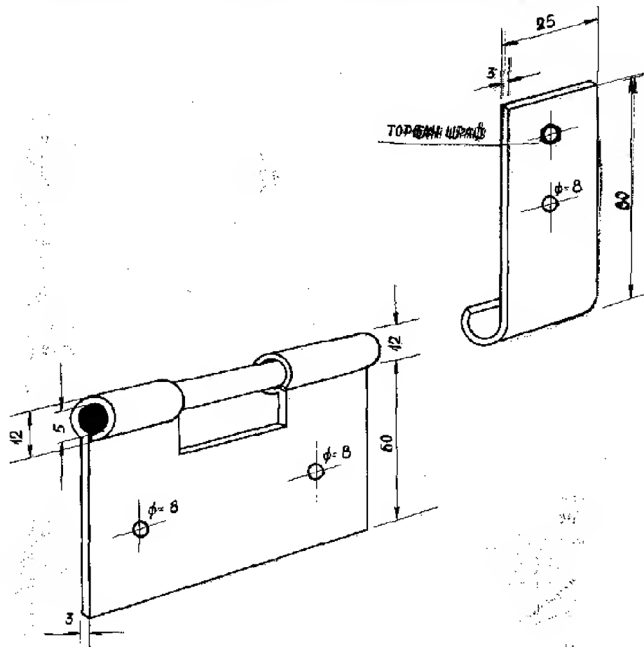
Шарке за Дадан-Блатове кошнице и полошке
